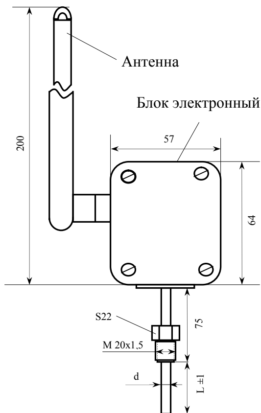
Рисунок 1 - Размеры термометра с аналоговым преобразователем Pt 1000
